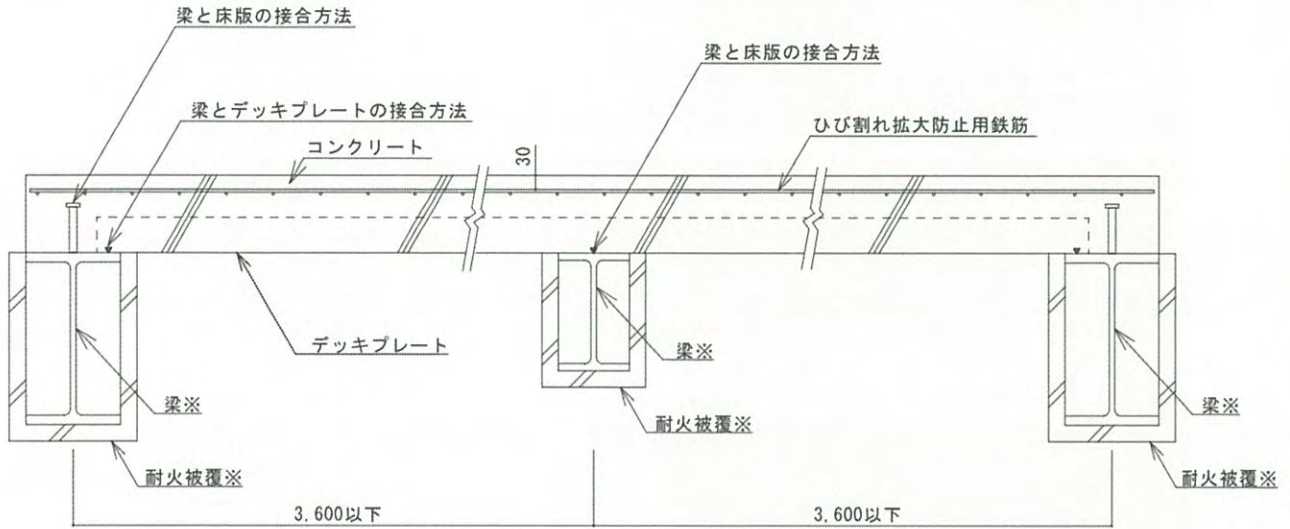
A-A 断面図
