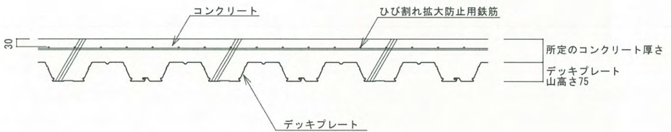
B-B 断面図
